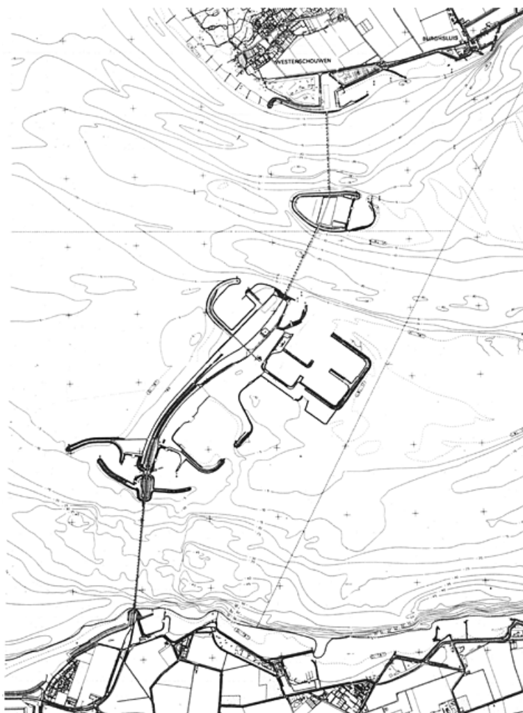
Stormvloedkering Oosterschelde
