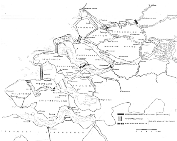
Deltawerken, schema afsluitingen
